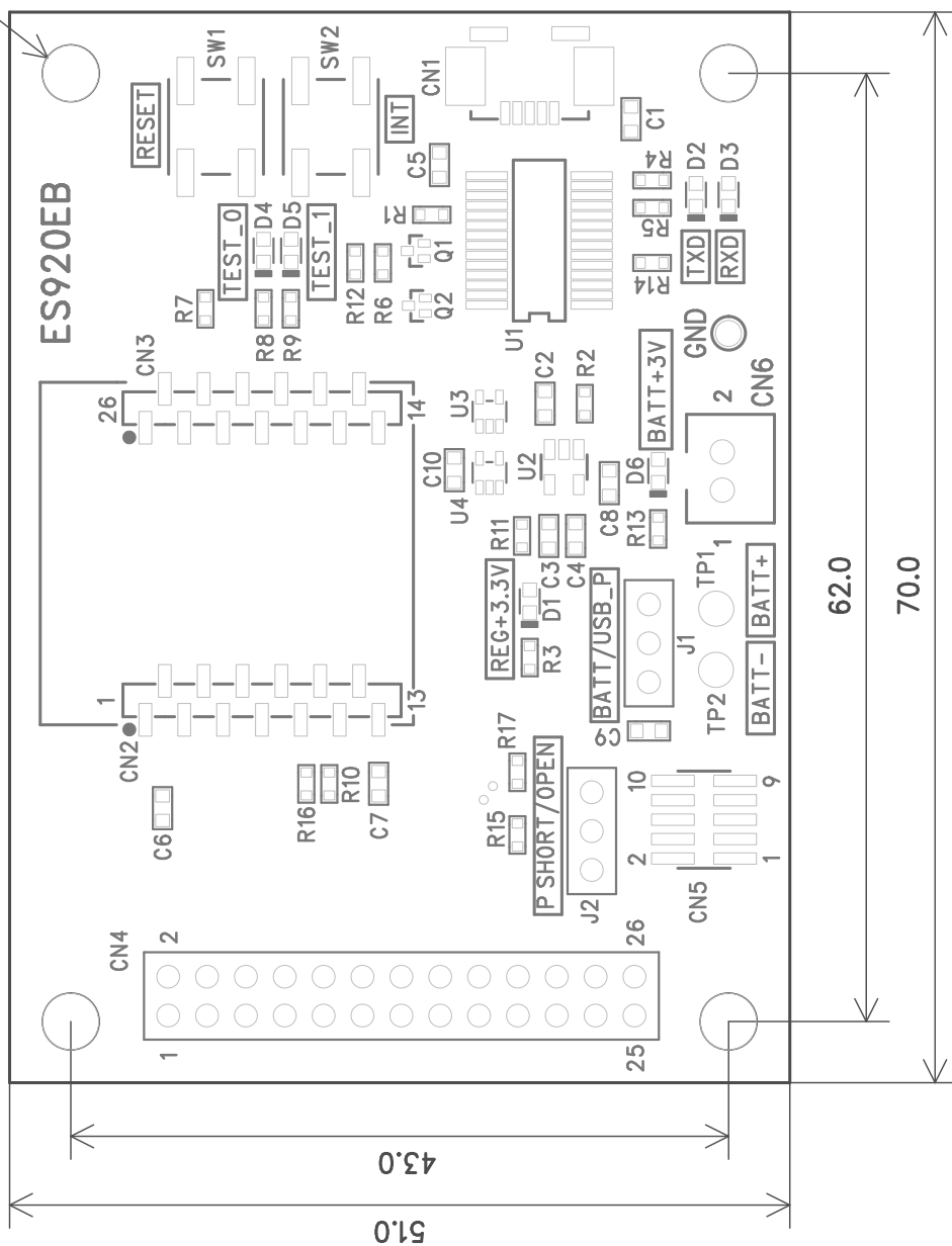
ES920EB寸法図 SCALE 2:1
