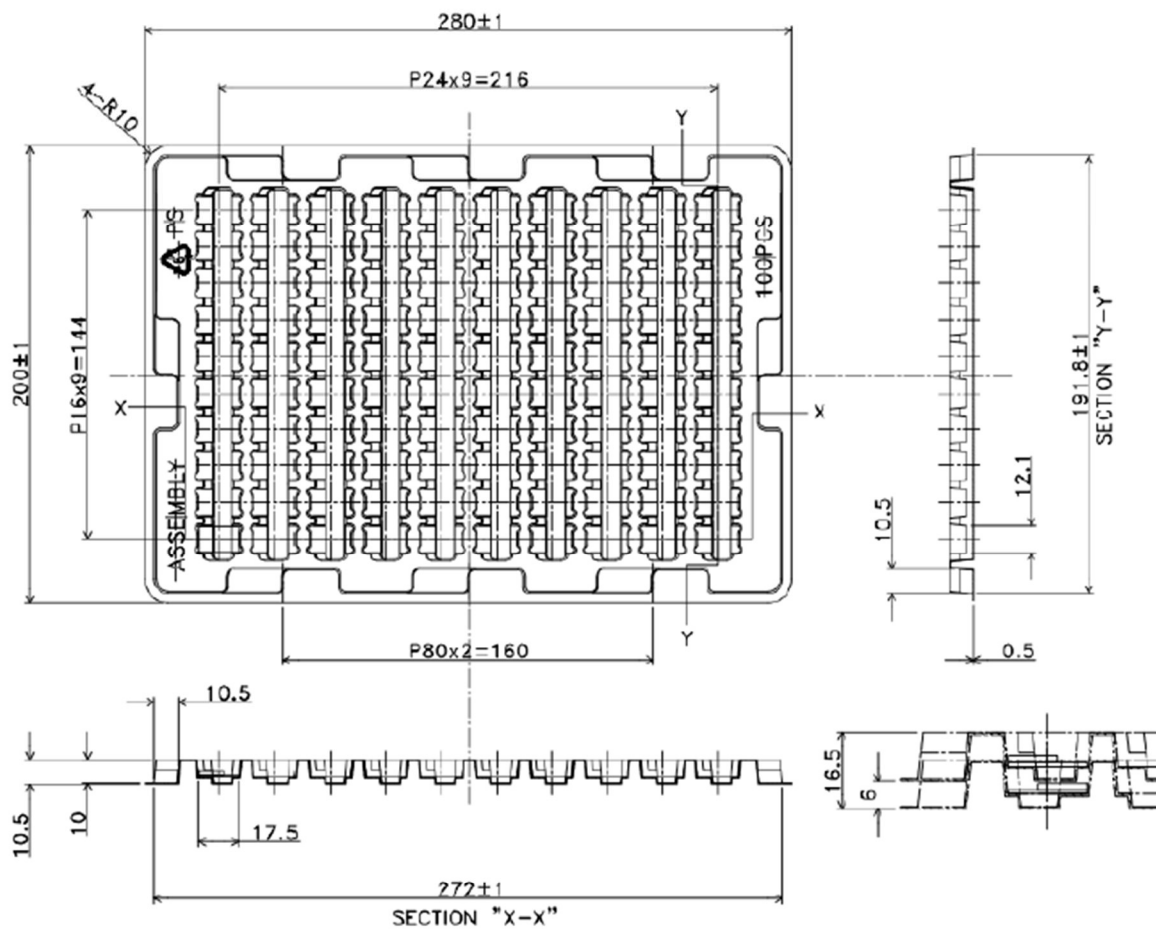
■トレイ寸法図
