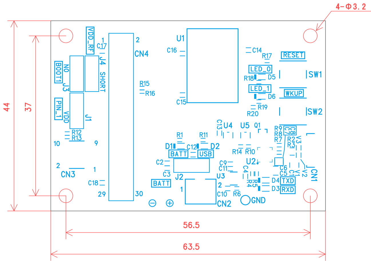
ES920LR3EB 寸法図 SCALE 2:1
