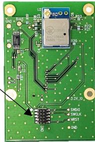
デバッグ用コネクタ
