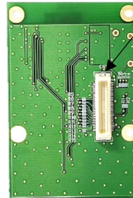
Armadillo 接続用コネクタ
