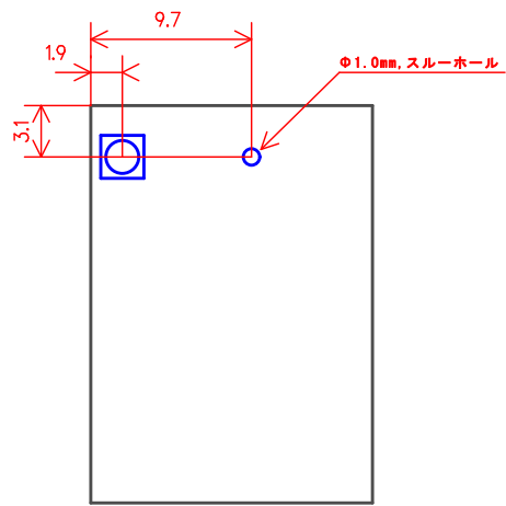
アンテナ位置寸法図
