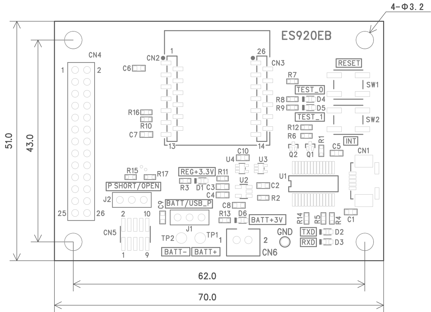
ES920EB寸法図
